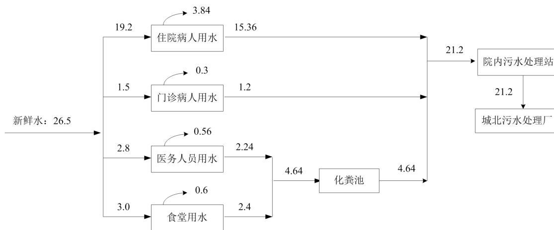
图 1-1 项目水平衡图（单位： \text{m}^3/\text{d} ）
