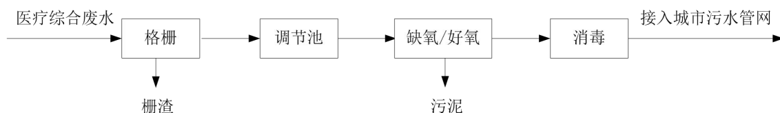
图 7-2 污水处理设施工艺流程图
